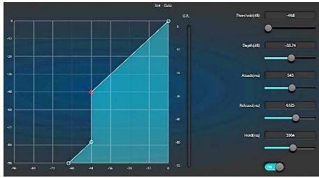
Модуль нойз-гейта (Noise Gate)
