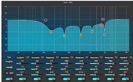
Модуль параметрич. EQ (5/8/12-Band)
